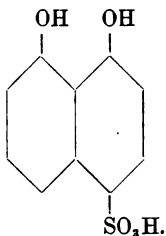
Dioxynaphtalinsulfosäure S.
